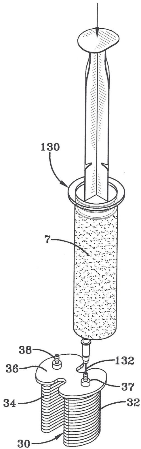
FIG-14A
